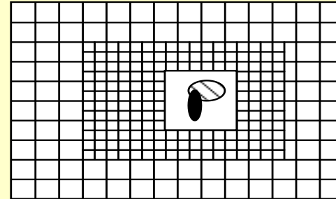
Busca Recursiva
