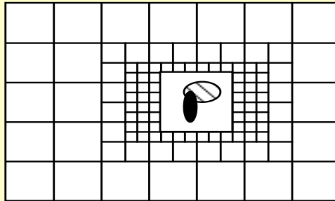
Busca Hierárquica
