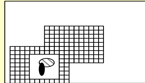
Busca Recursiva
