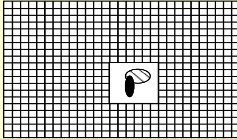
Busca Hierárquica
