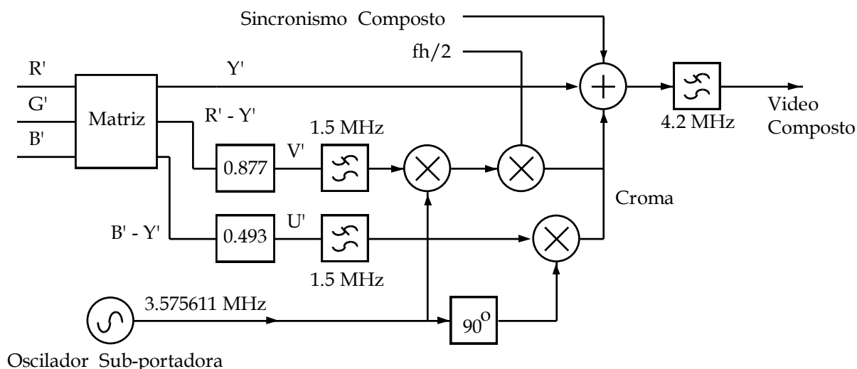
Fig. 8.1 - Modulador PAL-M
