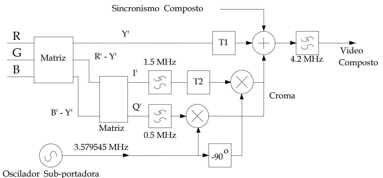
Fig. 7.1 - Modulador NTSC
