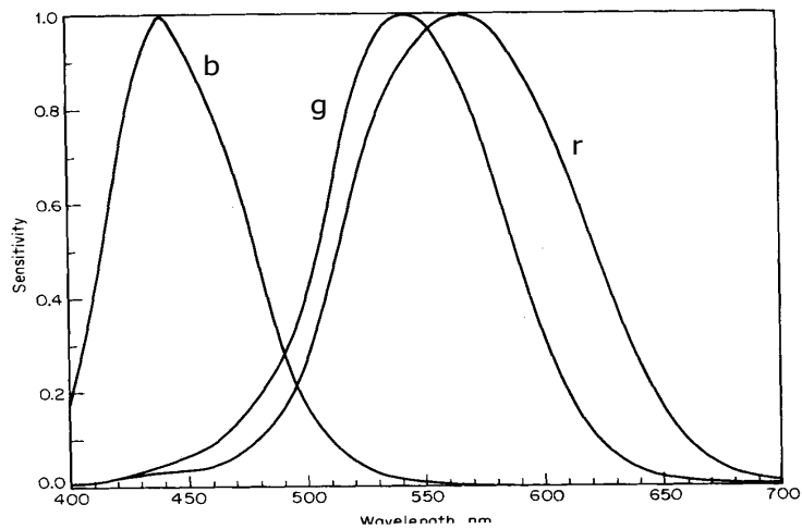
Fig. 2.2 - Sensibilidade espectral (médias, normalizada) para os três tipos de cones na retina humana
