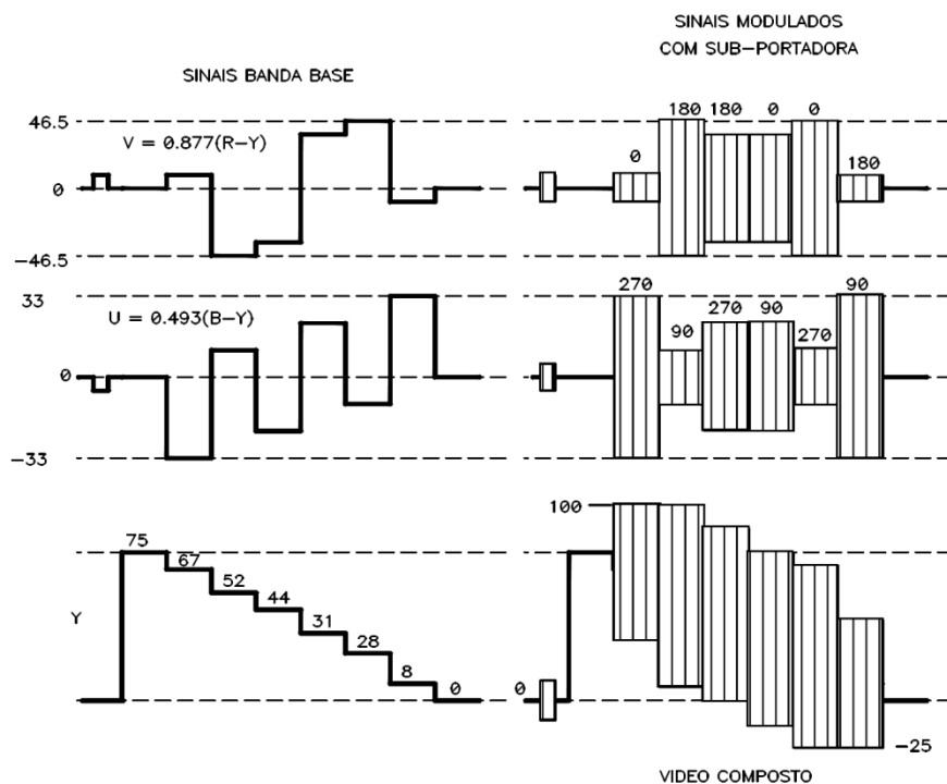
Fig. 8.2 - Formas de Onda no Modulador PAL-M (Padrão de Barras a 75% - amplitudes em IRE; fases em graus)
