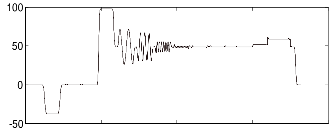
Efeito de intermodulação luma-croma (Filtro de rejeição de croma ativado):
