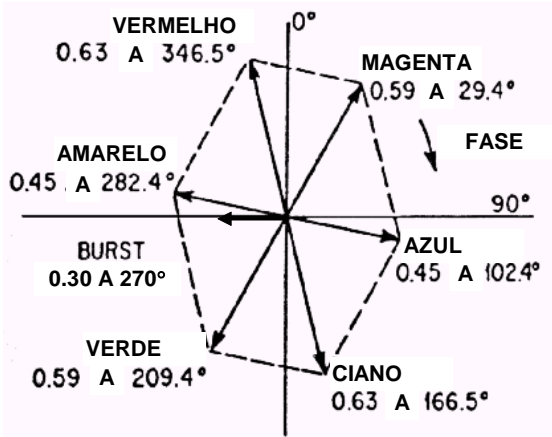
Fig. 7.2 - Diagrama Vetorial do Sinal de Crominância
