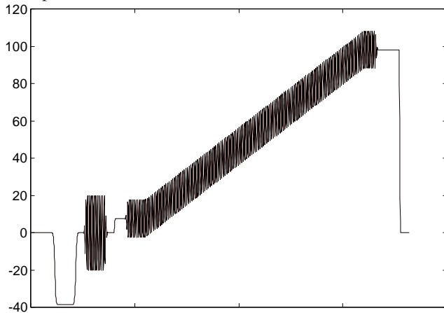
Rampa Modulada:
