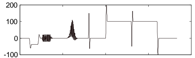
Atraso do sinal de croma:
