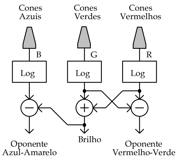
Fig. 2.1 - Modelo de Oponentes para Visão a Cores
