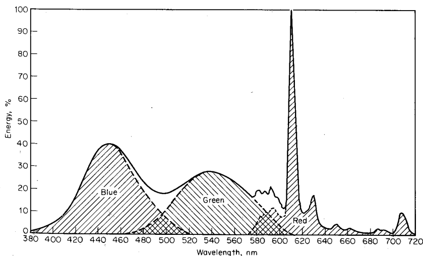
Fig. 4.2 - Densidade Espectral de Potência para Primários NTSC Típicos (para mesma densidade de corrente)
