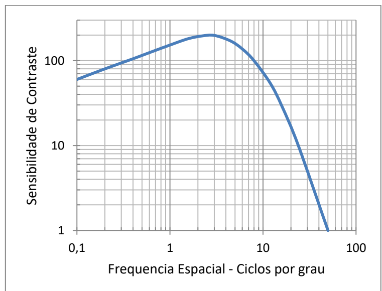
Fig. 3.2 - Função de Transferência de Modulação da Visão Humana
