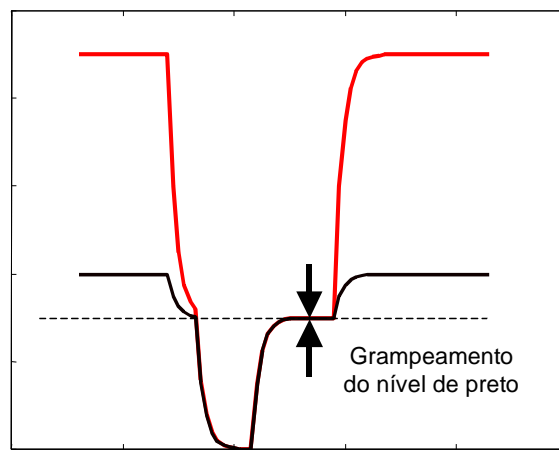
Fig. 7.6 – Acoplamento AC e Grampeamento no Pórtico Posterior
