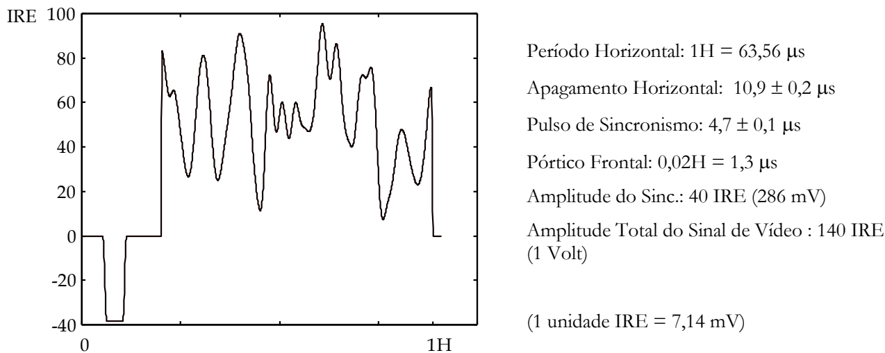
Fig. 6.1 - Sinal de Vídeo Composto (RS-170)
