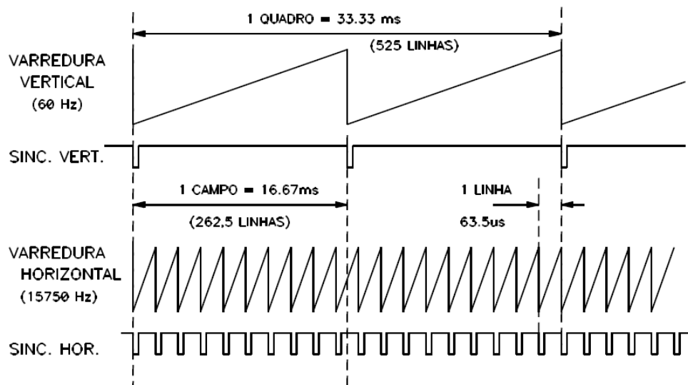
Fig. 5.1 - Varredura com Entrelaçamento
