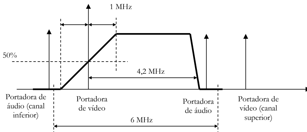
Fig. 11.1 - Modulação AM-VSB para Radiodifusão de TV
