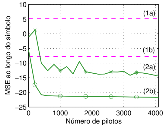
Fig. 8. Erro quadrático médio ao longo do símbolo OFDM: (1a) Sem estimação do canal para o Brasil A; (2a) Com estimação linear para o Brasil A; (1b) Sem estimação do canal para o Brasil D; (2b) Com estimação linear para o Brasil D.
