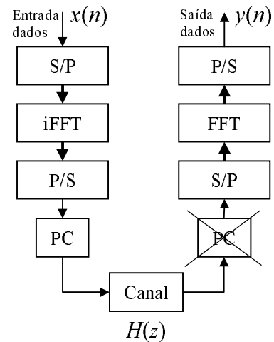
Fig. 1. Diagrama de blocos simplificado da transmissão e da recepção com OFDM.
