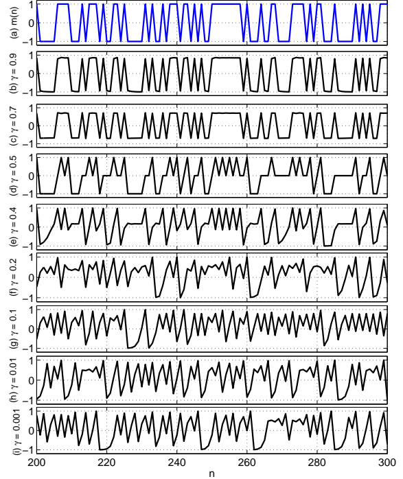
Figura 3: Sinais s(n) gerados a partir de uma mensagem m(n) utilizando-se o mapa quadrático e função de codificação c com diversos valores de \gamma : (a) mensagem m(n) (as amostras foram ligadas por segmentos de reta para facilitar a visualização); sinais s(n) com (b) \gamma = 0.9 , (c) \gamma = 0.7 , (d) \gamma = 0.5 , (e) \gamma = 0.4 , (f) \gamma = 0.2 , (g) \gamma = 0.1 , (h) \gamma = 0.01 e (i) \gamma = 0.001 .
