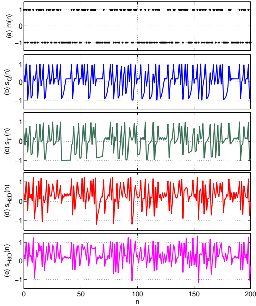
Figura 2: Sinais no transmissor do sistema da Figura 1 utilizando-se a função de codificação da Eq. (10) com \gamma = 0.4 . Em todos os casos, considerou-se condições iniciais \mathbf{x}(0) nulas: (a) mensagem m(n) e sinais s(n) transmitidos usando (b) mapa quadrático, (c) mapa tenda inclinada, (d) mapa Hénon 2D e (e) mapa Hénon 3D.
